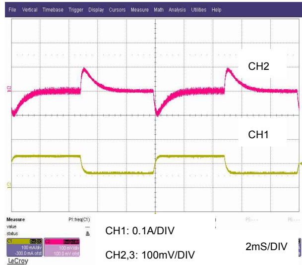
Vin=24V, Vo=12V@0.13A,At 25°C
